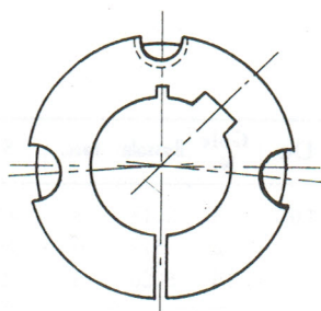
esecuzione A n° 3 fori
